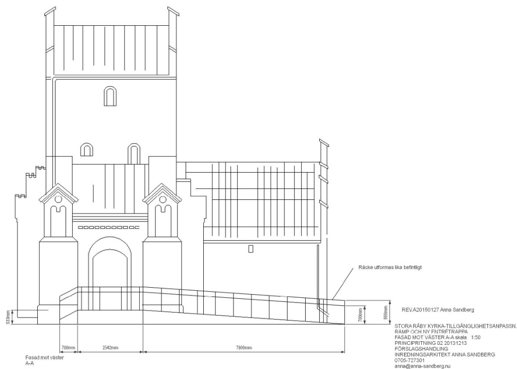
Figur 3. Ritning på tillgänglighetsanpassning vid Stora Råby kyrka, enligt bygghandlingarna.
